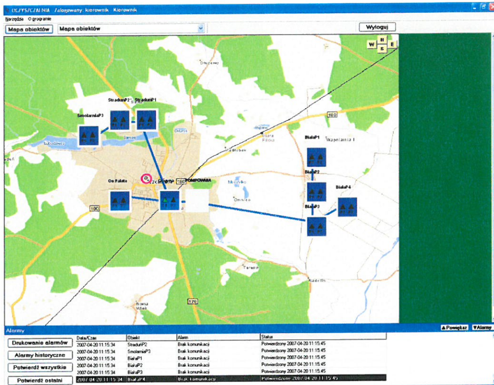
Główne okno synoptyczne wizualizujące monitorowane objekty.
